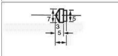
Vickers 136° Einsatz Briviskop
