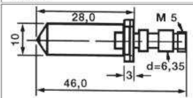
Vickers 136° Zwick 2
