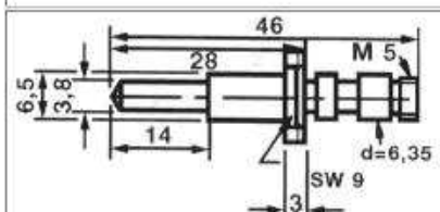
Rockwell 120° Sonderhalter
