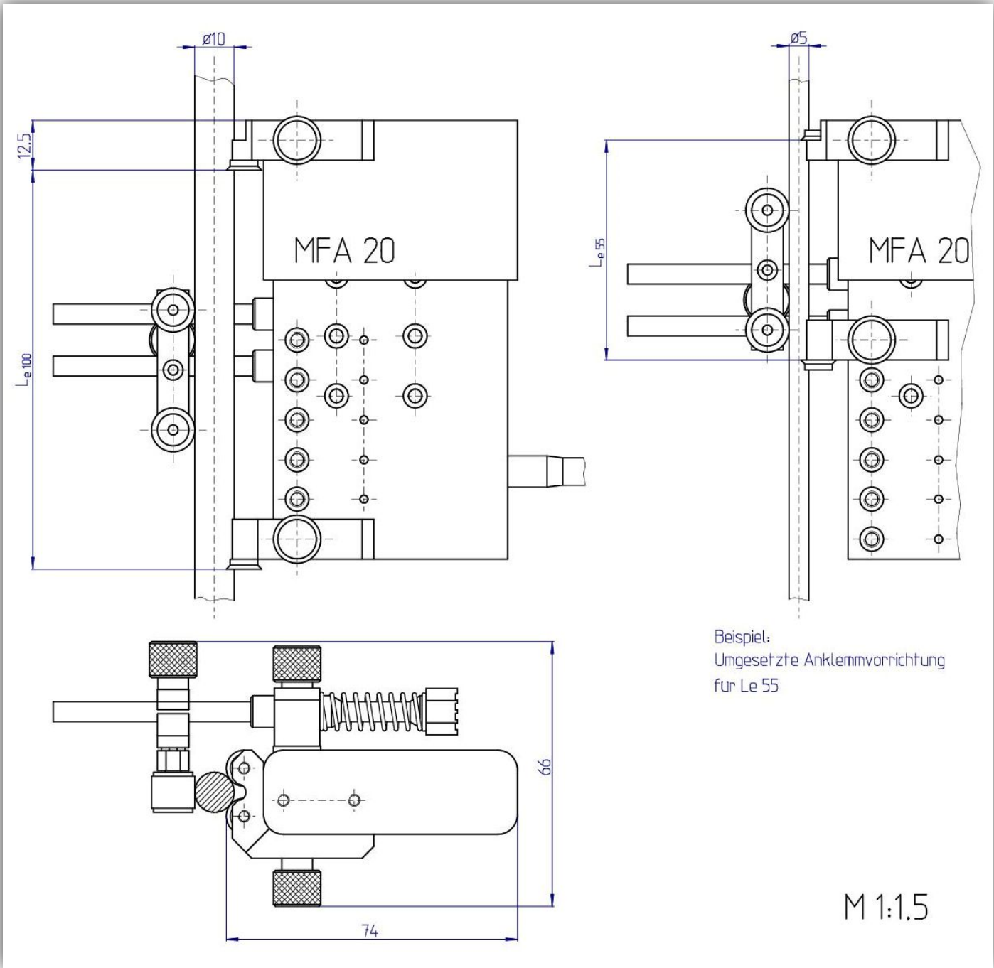
Bild 2: MFA 20 - Abmessungen
