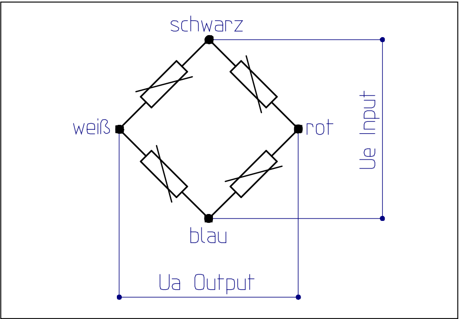
Bild 1: Prinzip-Schaltbild: DMS-Vollbrücke
