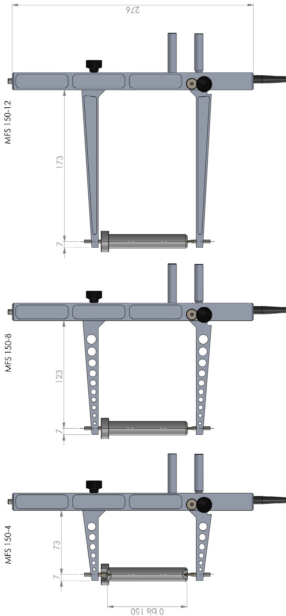
Zeichnung 1: MFS 150 - 4 / 8 / 12 Abmessungen
